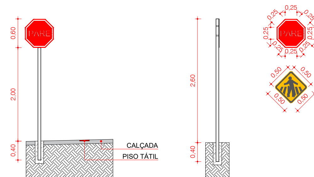
02 DETALHAMENTO DO SUPORTE DA PLACA ESC.: 1/50
