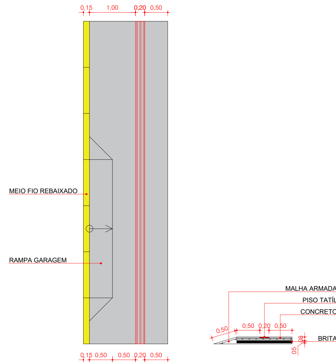
06 DETALHAMENTO DAS RAMPAS DE GARAGEM ESC.: 1/50
