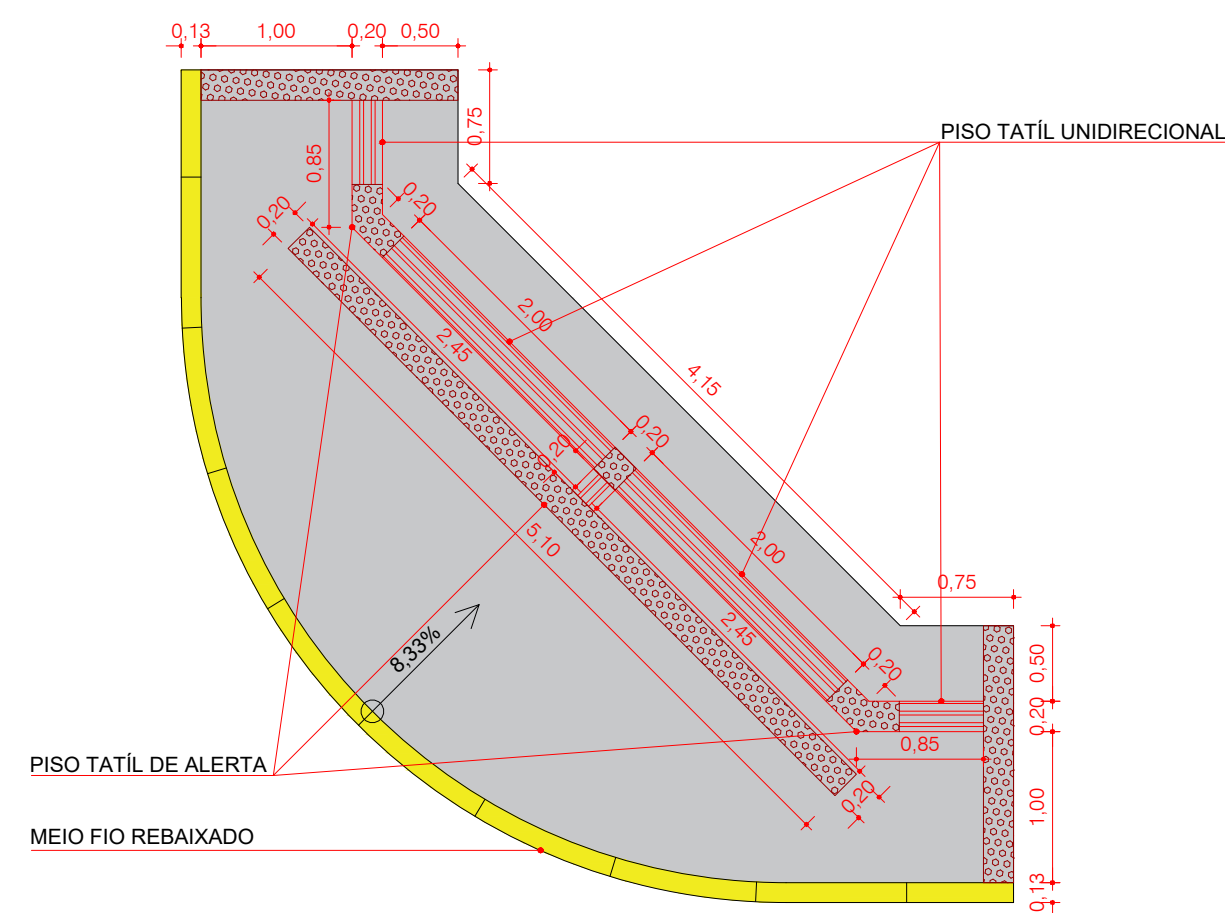
04 DETALHAMENTO DAS RAMPAS DE ESQUINA ESC.: 1/50
