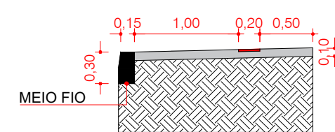
01 DETALHAMENTO PASSEIO ESC.: 1/50
