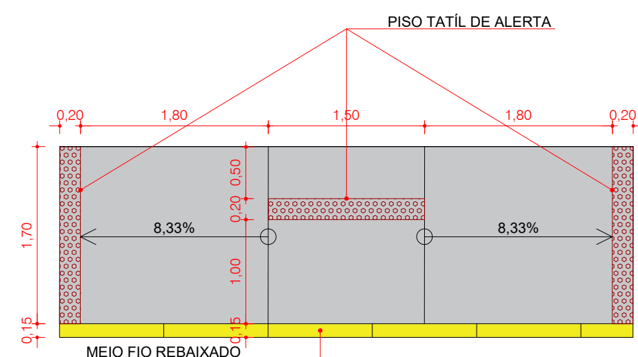
05 DETALHAMENTO DAS RAMPAS ESC.: 1/50
