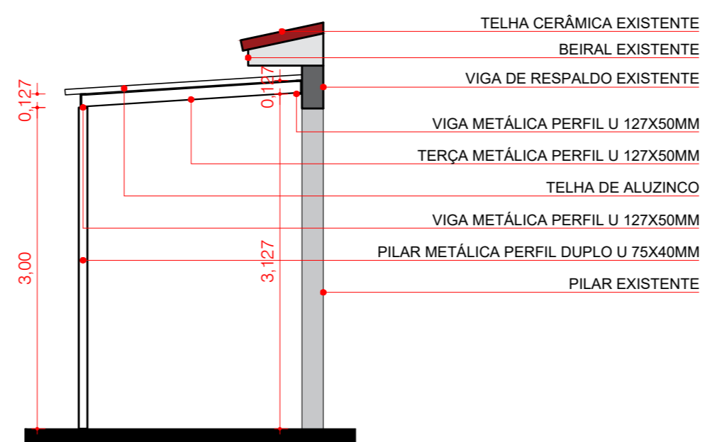
07 CORTE BB" ESC.: 1/50
