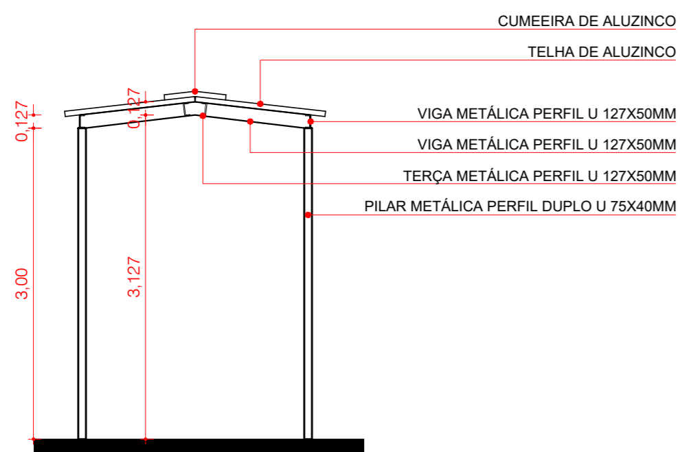
06 CORTE AA" ESC.: 1/50
