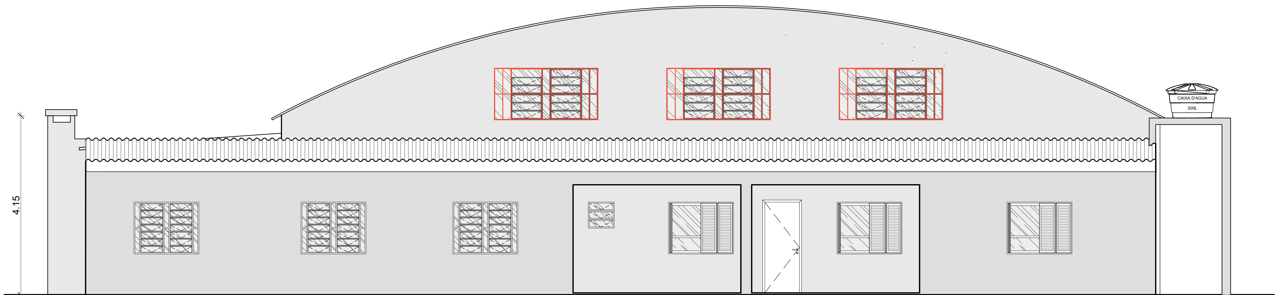
04 VISTA SUL Fachada Agroindústria Esc.: 1/50
