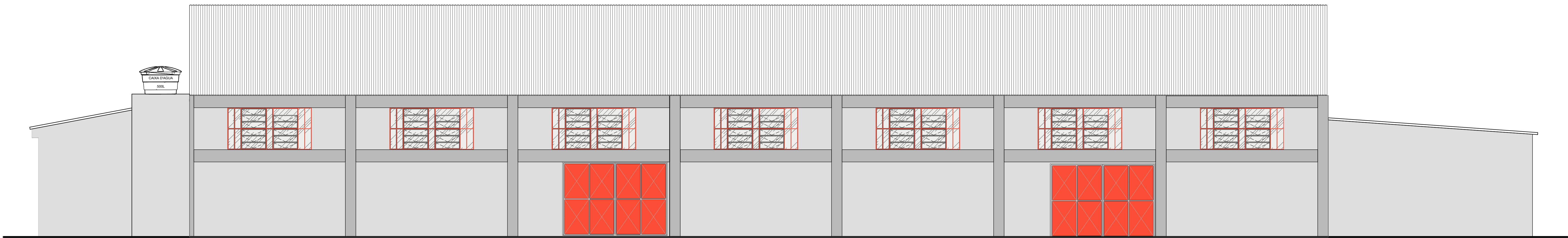
03 VISTA OESTE Fachada principal Esc.: 1/50
