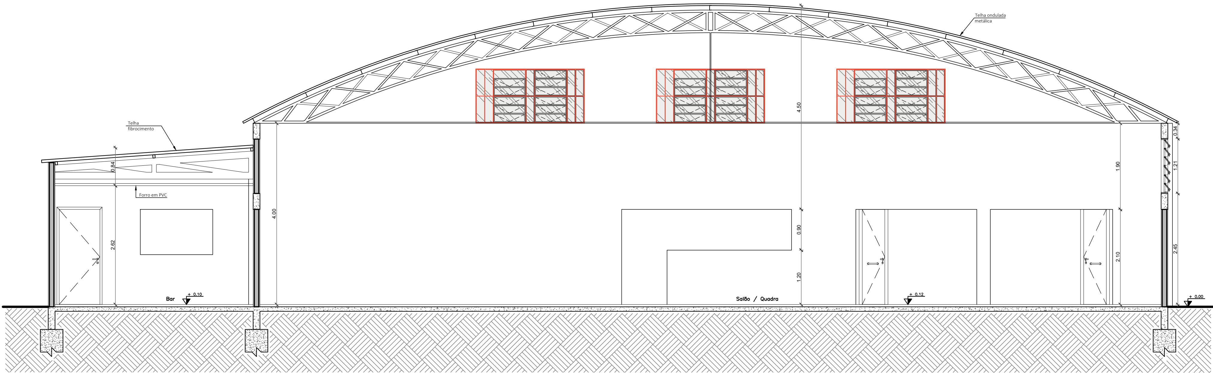
01 CORTE AA Esc.: 1/50
