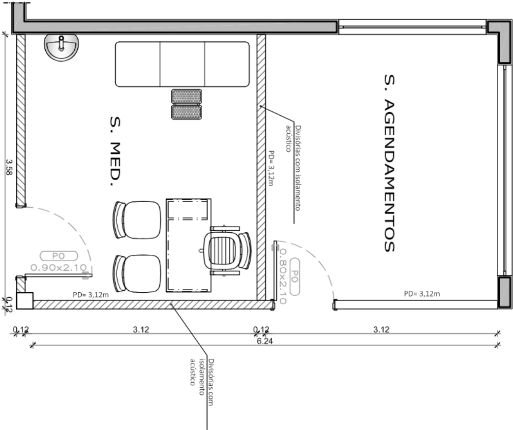
02 PLANTA BAIXA PRETENDIDA ESC.1/50
