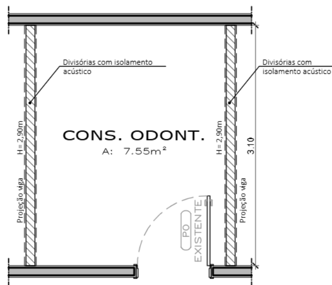
04 PLANTA BAIXA PRETENDIDA ESC.1/50
