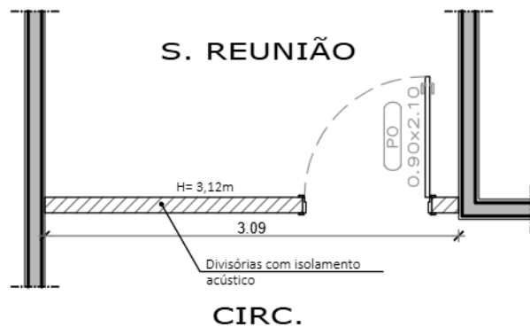
01 PLANTA BAIXA PRETENDIDA ESC.1/50
