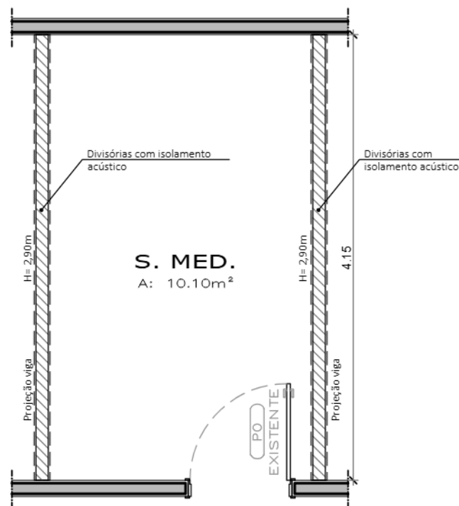
03 PLANTA BAIXA PRETENDIDA ESC.1/50
