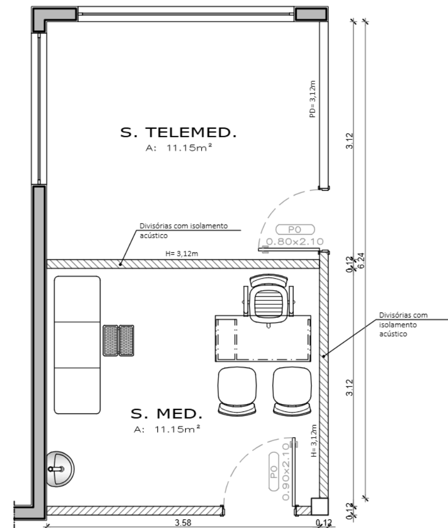
02 PLANTA BAIXA PRETENDIDA ESC.1/50
